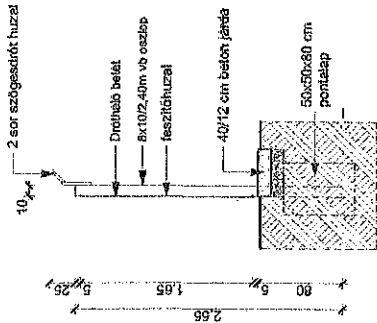
A-A METSZET M=1:50
